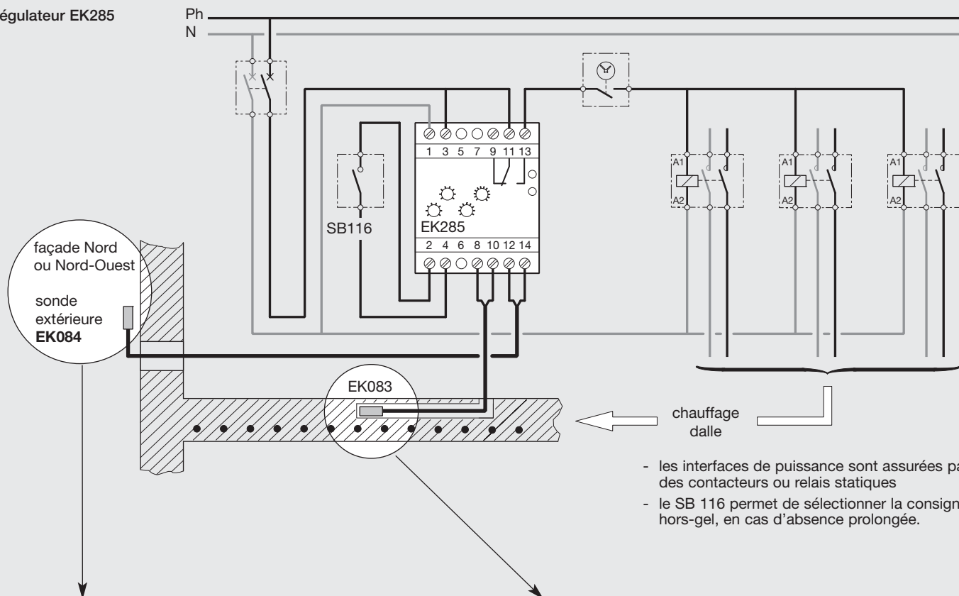
trame chauffante
