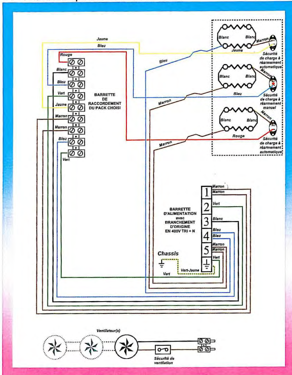
6-3-1 Schéma électrique de l'Accumulateur ACCURO
