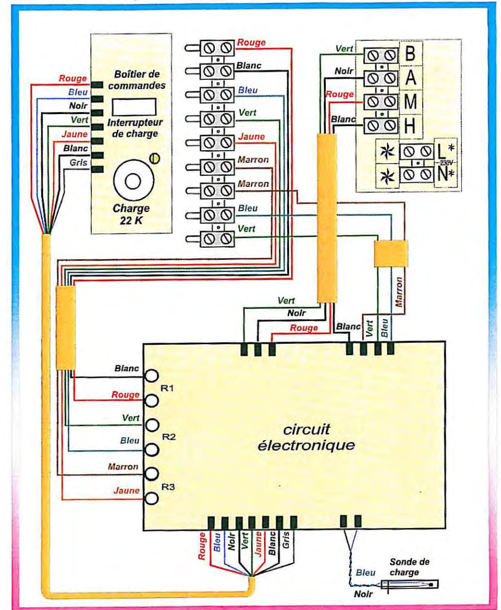
6-3-2 Schéma électrique du pack "Initial"
