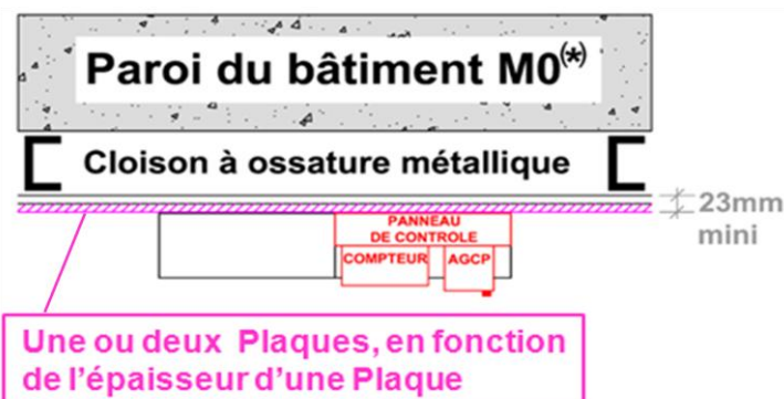
Schéma 5 : Cas N°3 Panneau de contrôle fixé sur plaque de doublage avec deuxième plaque de plâtre
