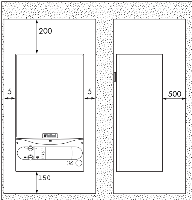
Fig. 3.3 Espaces de montage nécessaires Afb. 3.3 Vereiste vrije montageruimte Abb. 3.3 Erforderliche Montagefreiräume
