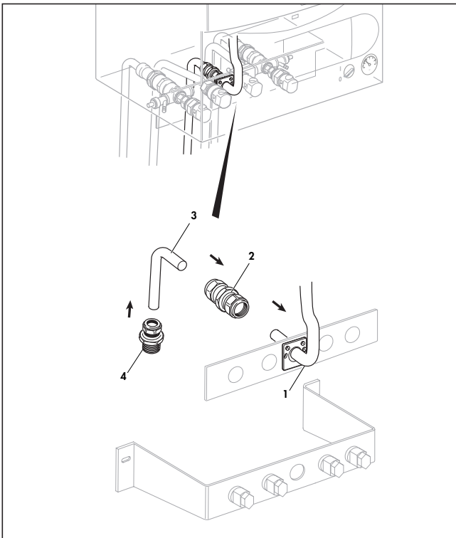
Fig. 3.7 Montage du raccord de gaz
