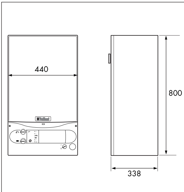
Fig. 3.4 Dimensions de l'appareil Afb. 3.4 Afmetingen van de gaswandketel Abb. 3.4 Geräteabmessungen
