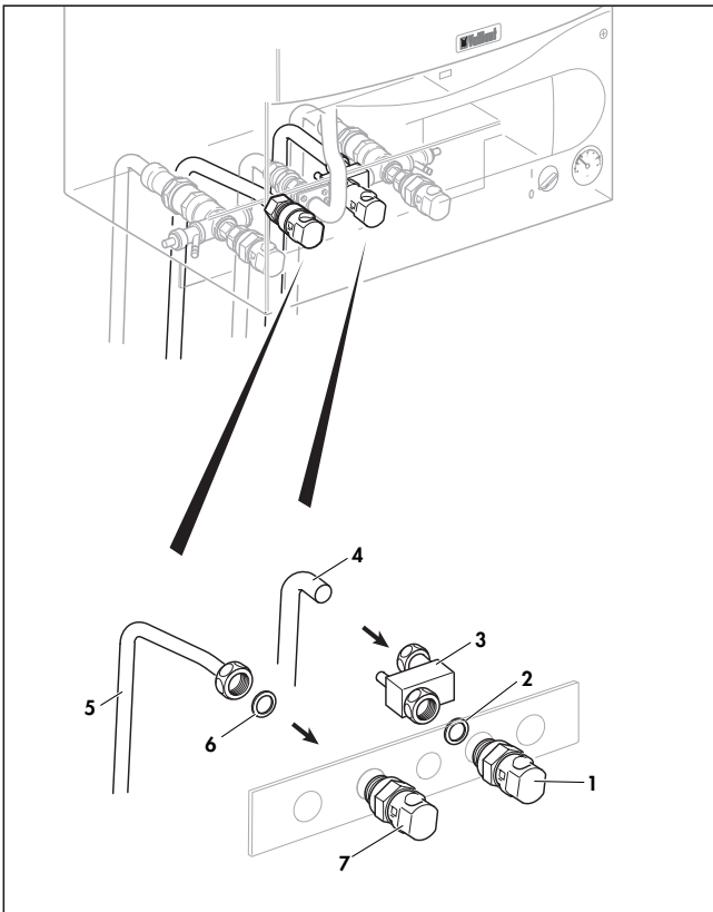
Fig. 3.8 Montage des raccords d'eau froide et d'eau chaude Afb. 3.8 Koud- en warmwateraansluiting monteren Abb. 3.8 Kalt- und Warmwasseranschluss montieren
