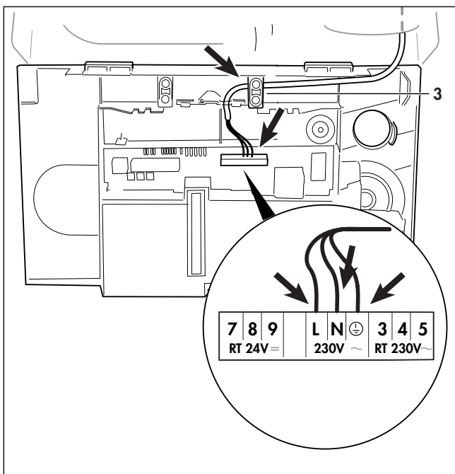
Fig. 3.12 Câblage Afb. 3.12 Kabeldoorvoering Abb. 3.12 Kabelführung
