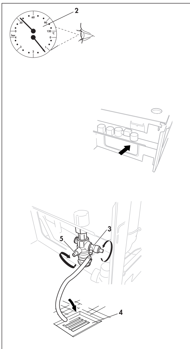
Fig. 7.3 Remplir et vider la chaudière
