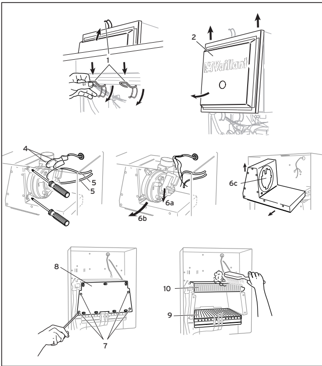
Fig. 7.1 Nettoyage du brûleur et de l'échangeur primaire Afb. 7.1 Reiniging van brander en primaire warmtewisselaar Abb. 7.1 Brenner und Primärwärmetauscher reinigen
