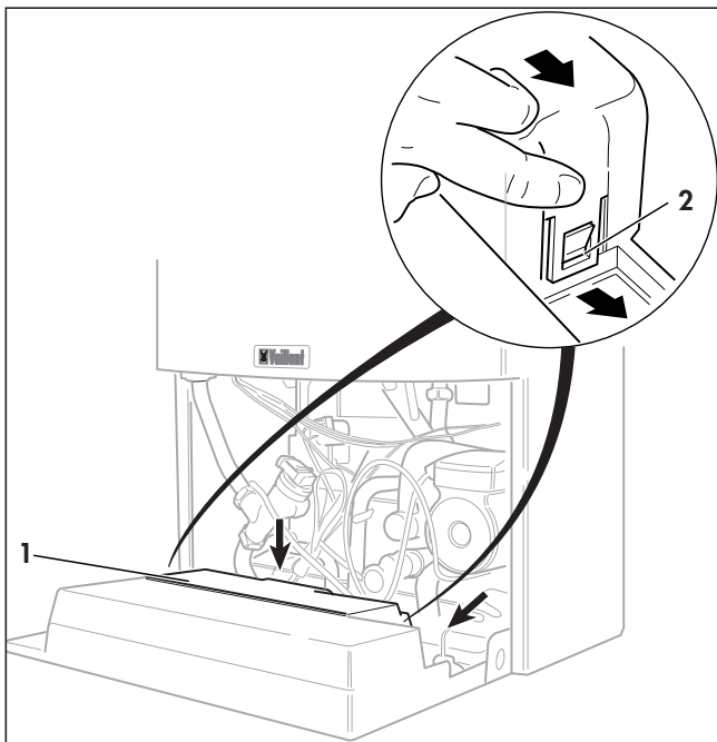
Fig. 3.11 Ouverture du dos du tableau de commande Afb. 3.11 Achterwand van het bedieningsbord openen Abb. 3.11 Schaltkastenrückwand öffnen
