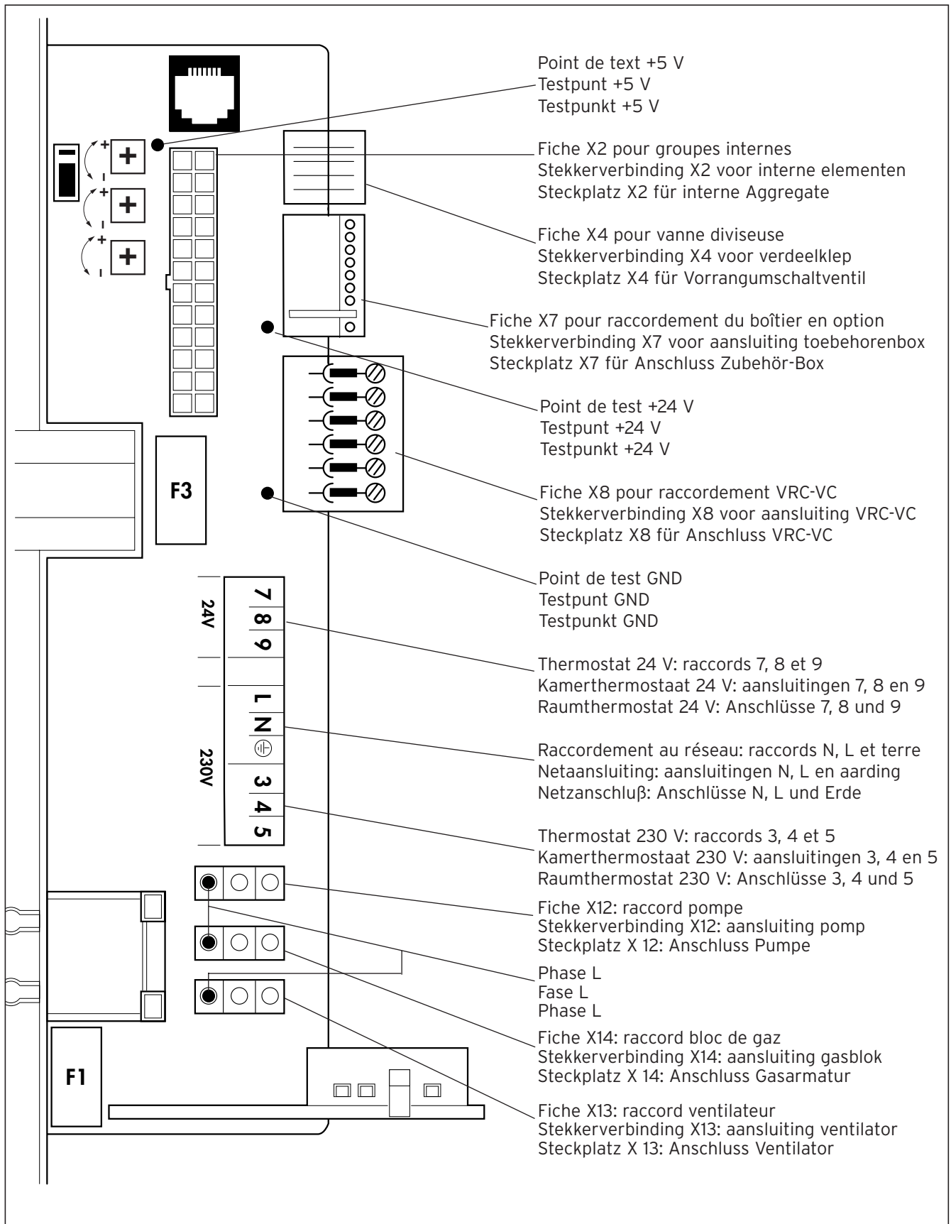
Fig. 3.13 Câblage des raccords
